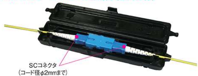
光コネクタスリーブ MS1 の適用例 (屋内仕様)
